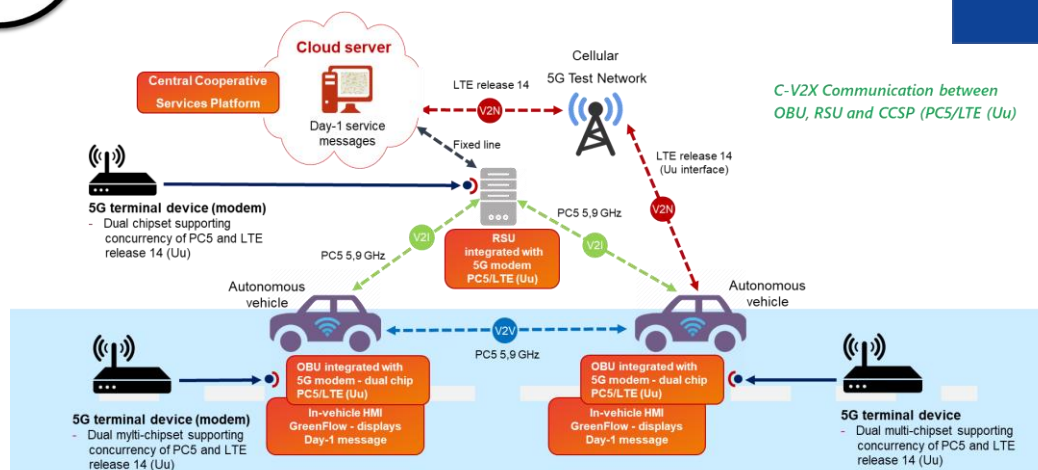
VTT - 5G test site Espoo, Finland
